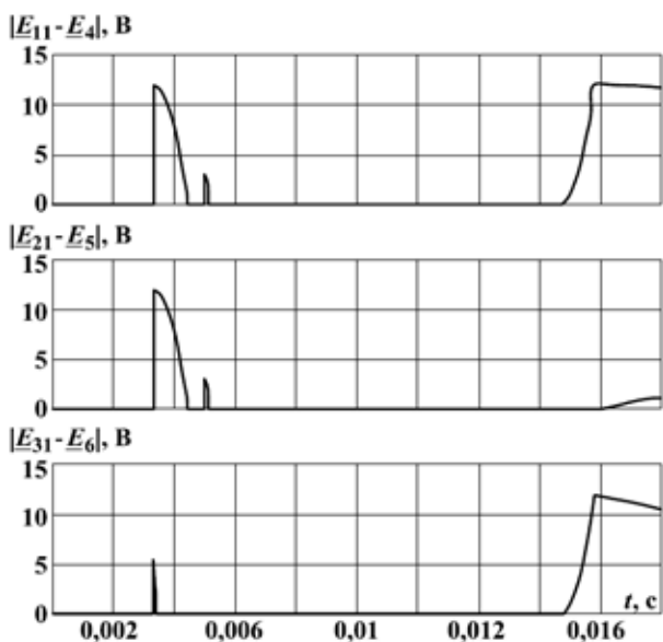
Рисунок 3 – Разности ЭДС при обрыве диода 4
