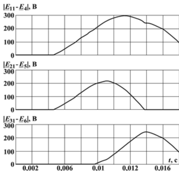
Рисунок 2 – Разности ЭДС при пробое диода 4
