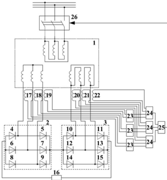
Рисунок 1 – Функциональная схема устройства защиты
